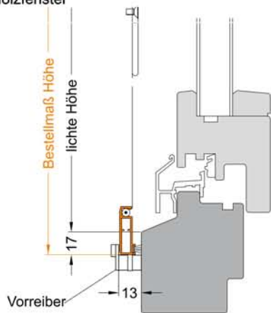
bei Holzfenster
