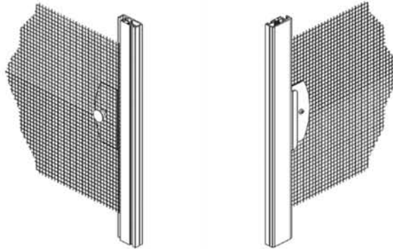
Ansicht innen Knopfgriff mit Innengewinde (10 615 999 07) und Kunststoffplatte (10 699 001 08 ...)
