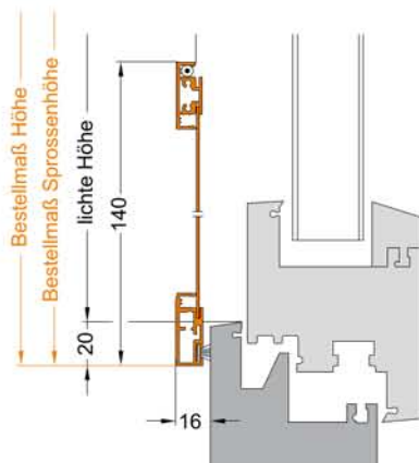
bei flächenversetzter Kunststoffür
