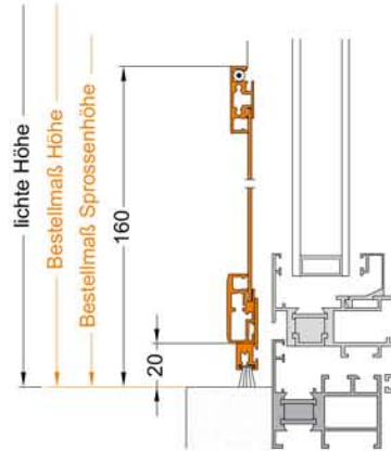
bei flächenbündiger Alutür
