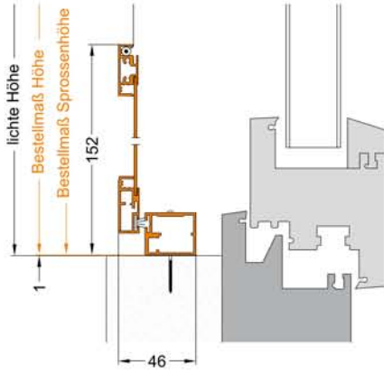
bei flächenversetzter Kunststoffür
